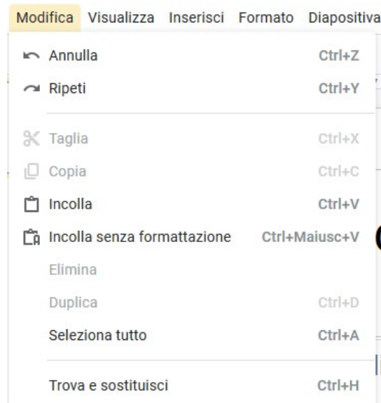
Figura 1: Menu Modifica
