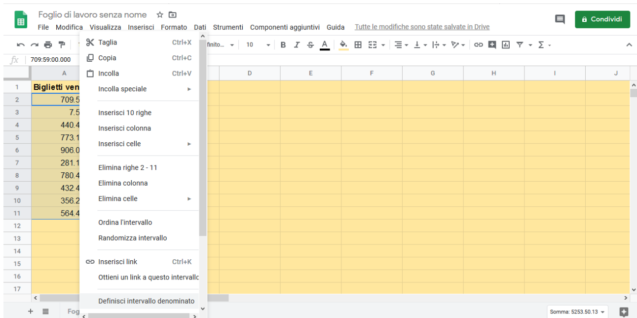
Figura 1: Definire intervallo
