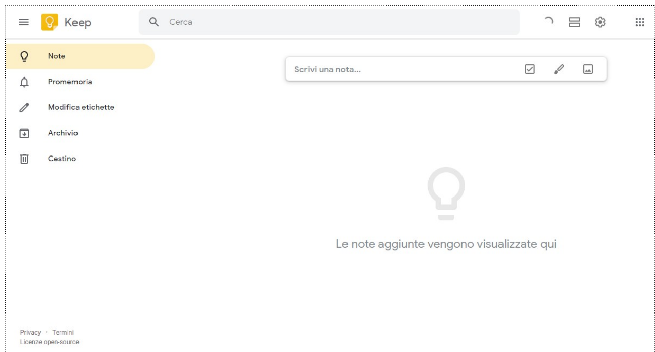
Figura 1: Interfaccia Keep
