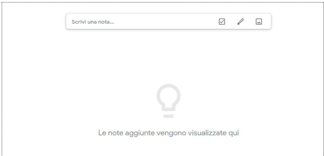
Figura 3: Spazio centrale
