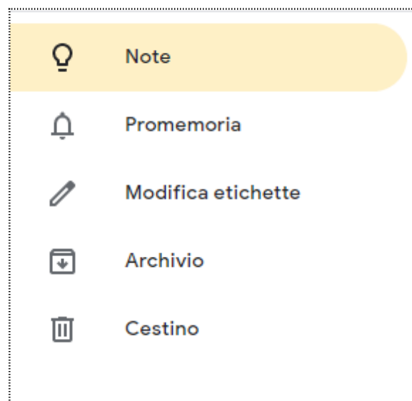
Figura 4: Barra laterale
